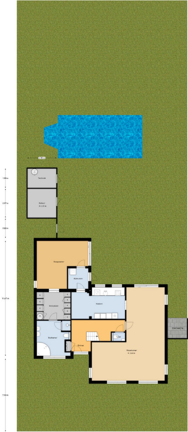
Begane grond
