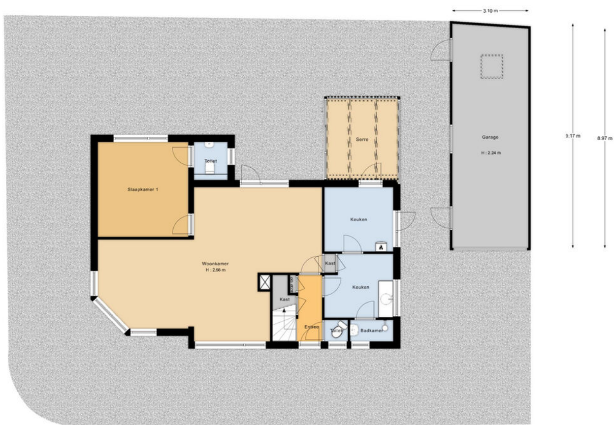
Begane grond overzicht
