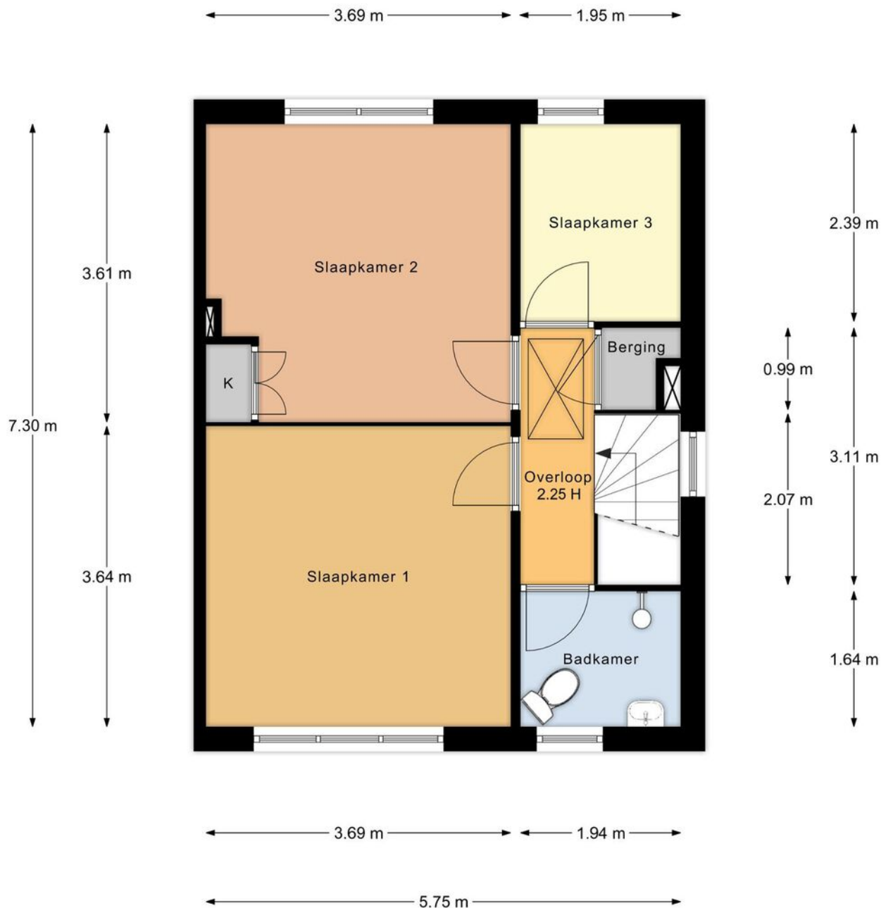
Eerste verdieping
